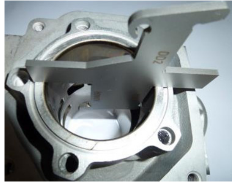
5.5.6 Egzoz portu zamanlaması (Silindir ID Tanımlama Kodu 223994, 223993, 613933)
